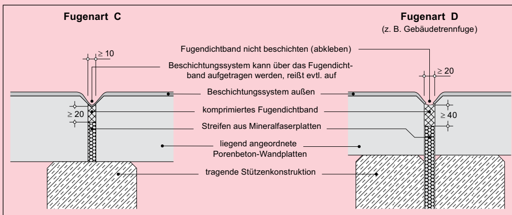
Abb. 11: Horizontalschnitte Fugenarten C und D - Abdichtung mit komprimiertem Fugendichtband
