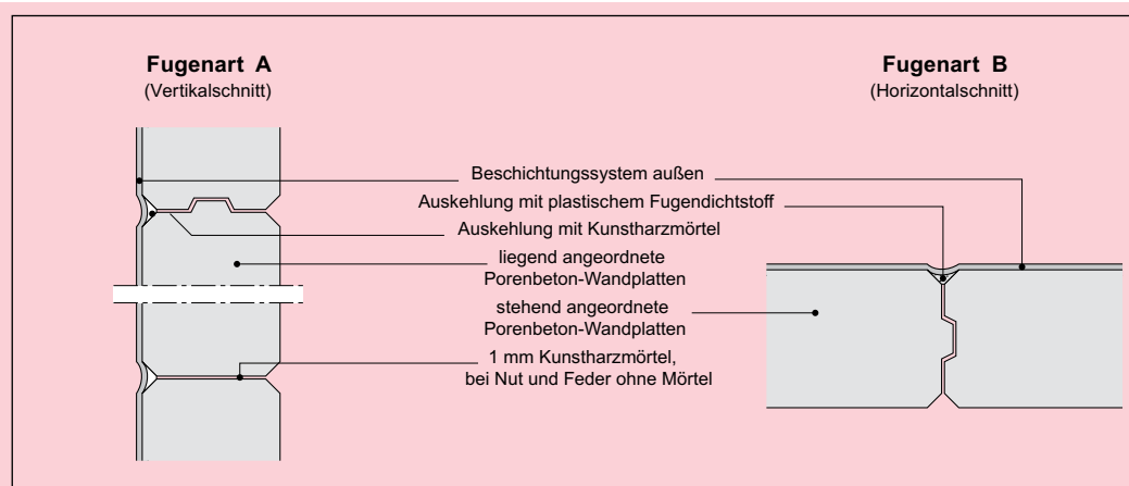
Abb. 9: Fugenarten A und B bei Horizontal- und Vertikalfugen - Ausgekehlt mit Kunstharzmörtel bzw. plastischem Fugendichtstoff
