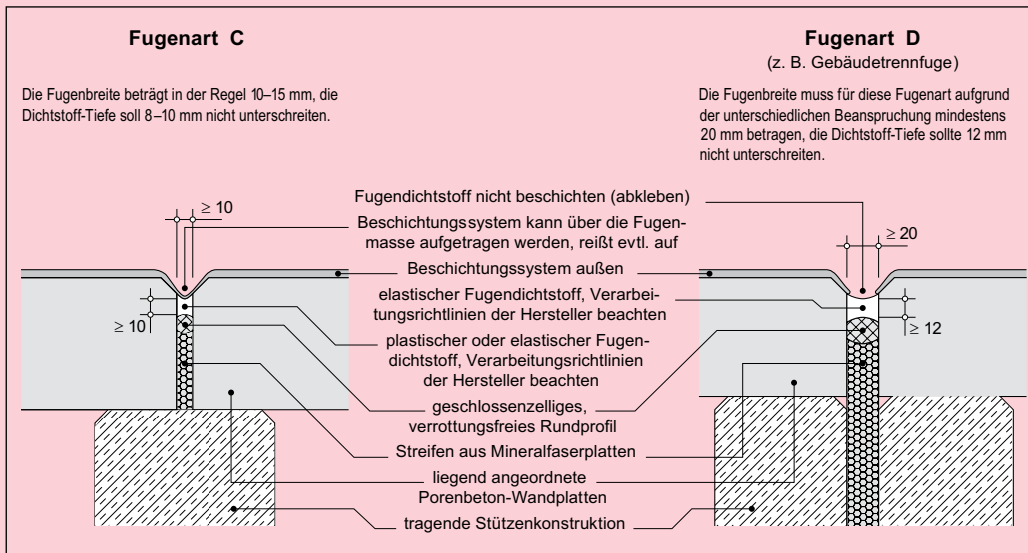
Abb. 10: Horizontalschnitte Fugenarten C und D - Abdichtung mit Fugendichtstoff
